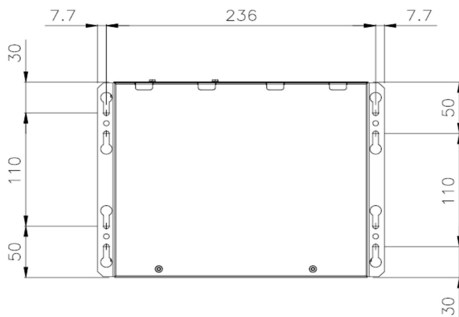
VISTA CONNETTORI
