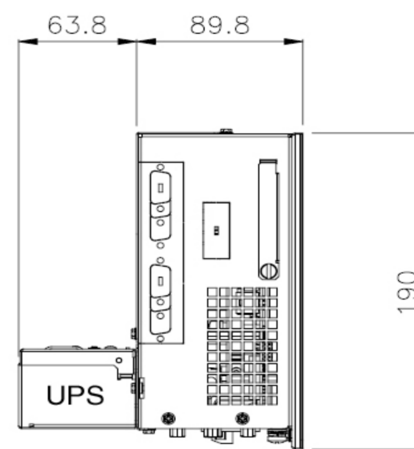
VISTA LATERALE
