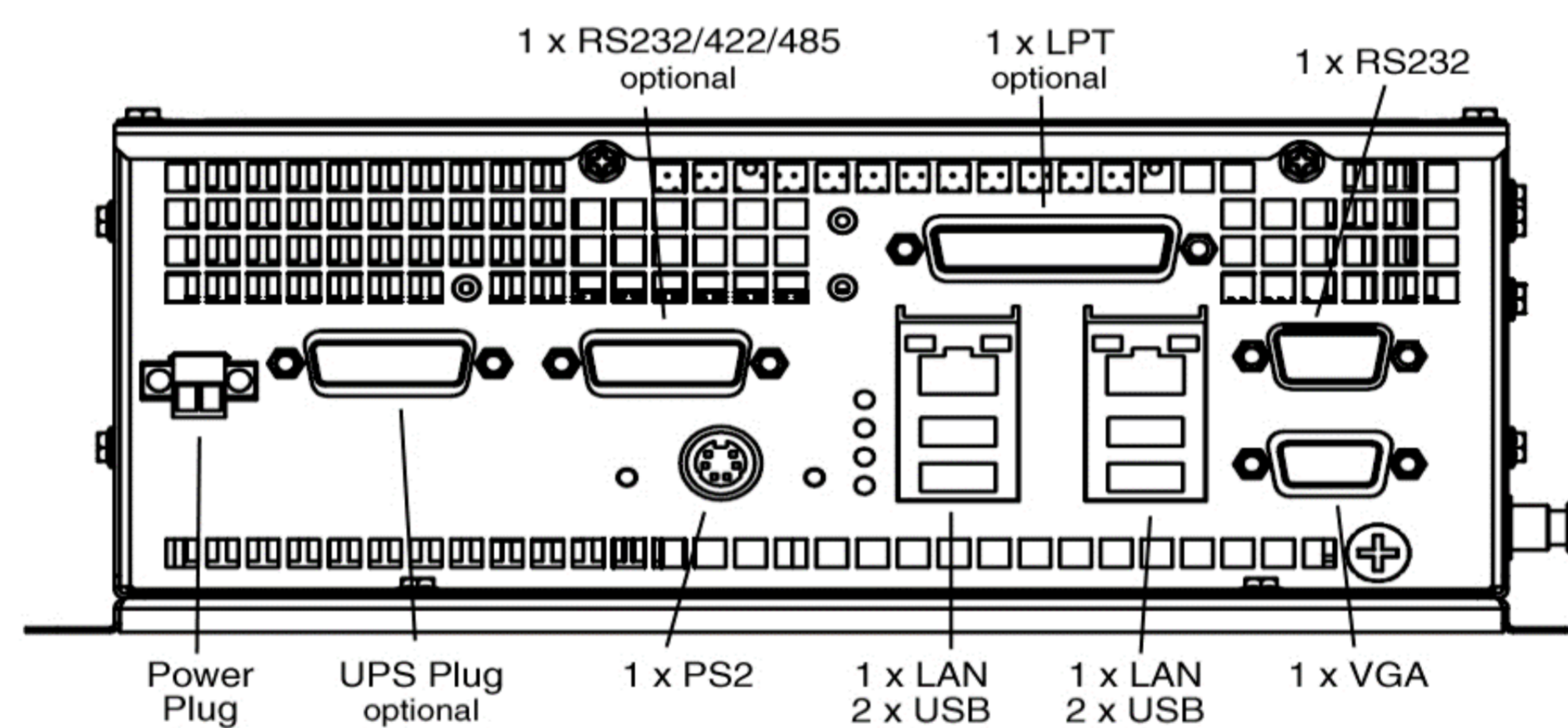
VISTA CONNETTORI
